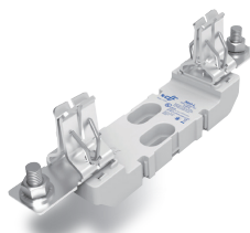
NH gPVシリーズ ヒューズベース/ヒューズリンク
