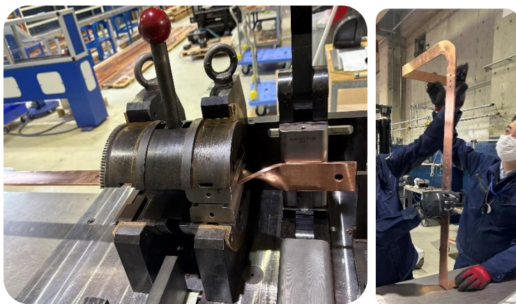
ツイスト曲げ加工・エッジワイズ曲げ加工
